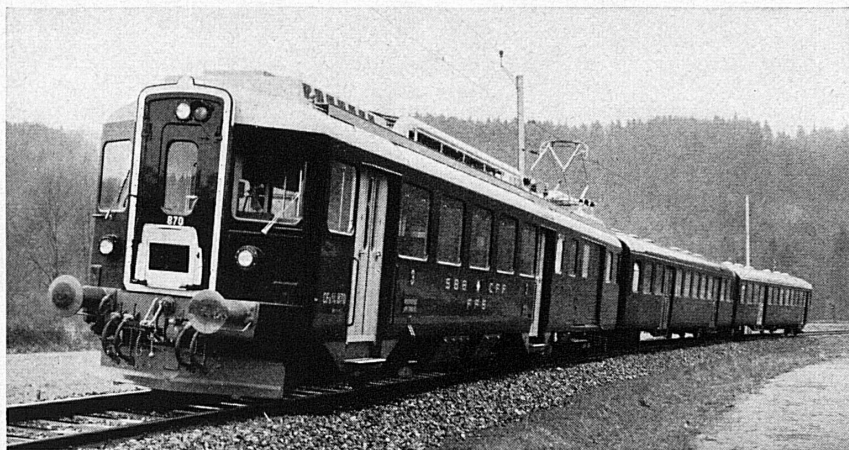
SBB-Pendelzug bestehend aus Triebwagen CFe4/4, Zwischenwagen C4ü und Steuerwagen BCt4ü
