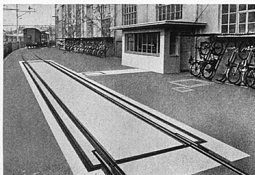
Brückenwaage für Geleisefahrzeuge. Wägefähigkeit 150 000 kg, Brückenlänge 16 m.
