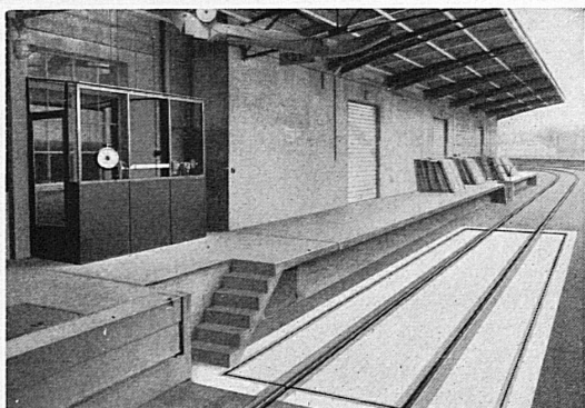
Brückenwaage für Geleise- und Straßenfahrzeuge. Wägefähigkeit 80 000 kg, Brückenlänge 16 m.
