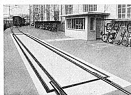
Brückenwaage für Geleisefahrzeuge. Wägefähigkeit 150 000 kg
