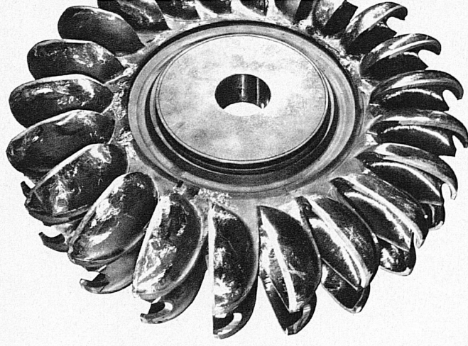
Eines der fünf an die Ateliers des Charmilles S. A., Genf, gelieferten Peltonräder für das Kraftwerk Koyna (Indien) Werkstoff: Chromnickelstahl (13%) Gewicht: 10,5 t Leistung je Turbine: 105000 PS
