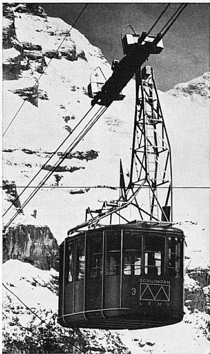
Telefonstation für Luftseilbahnen
