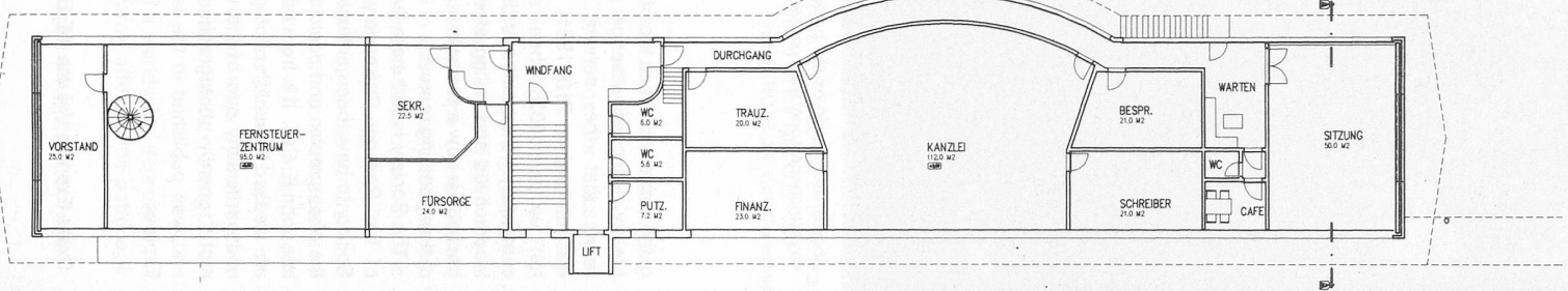
GRUNDRISS OG
