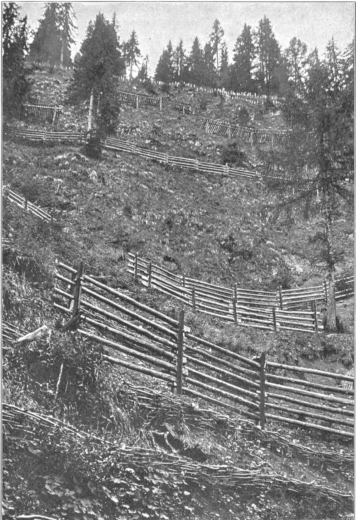
Parois protectrices et ponts à neige, élevés dans le couloir sud de l'avalanche de Calcestri près de Piotta.
