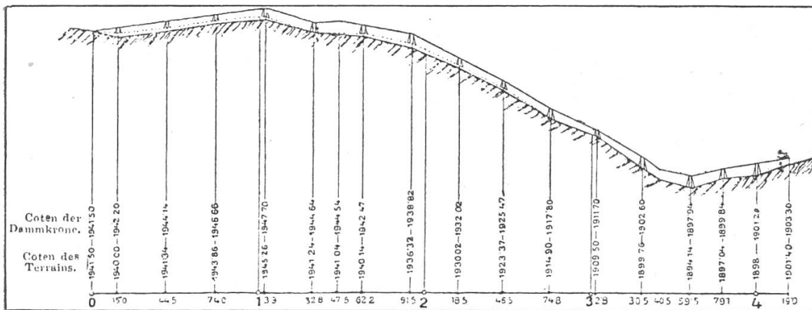
Fig. 3. Lawinen-Schuttdamm auf der Schmittenhöhe, Längenprofil.
