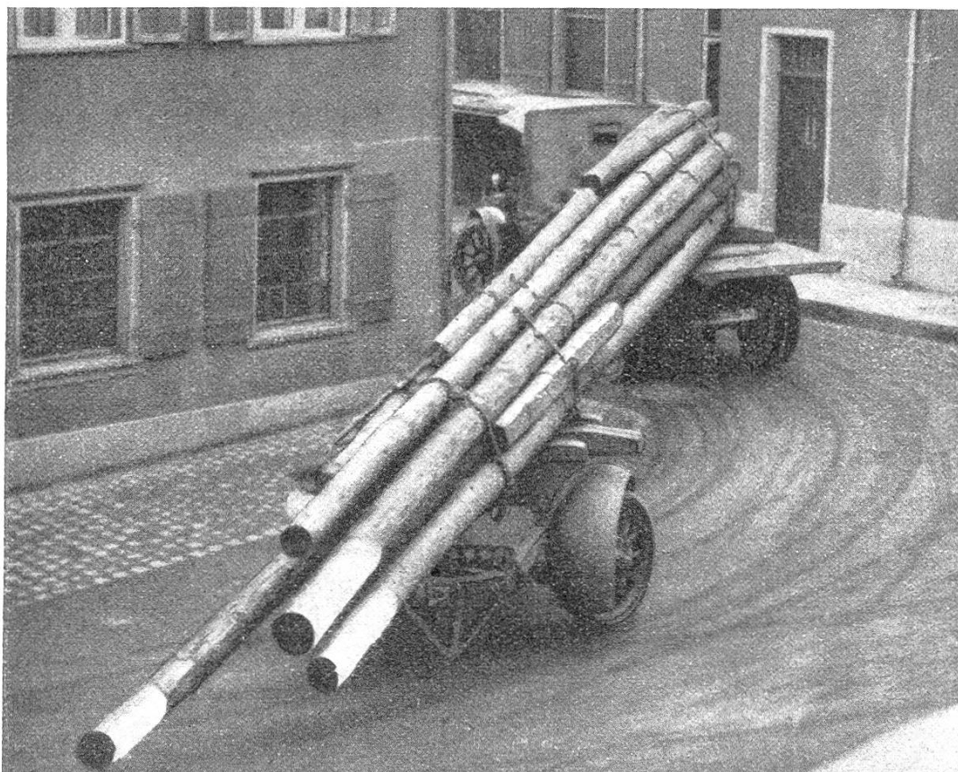
Saurer Langholztransportwagen. Der lenkbare Hinterwagen folgt der Spur des Vorderwagens und ermöglicht das Befahren scharfer Kurven.
