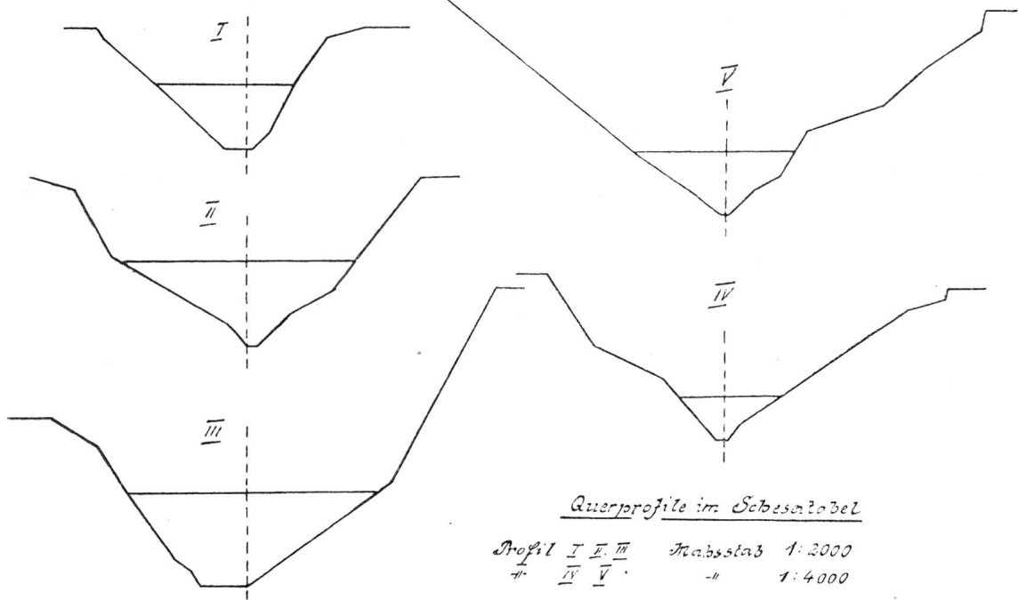
Abb. 5. Längen- und Querprofile des Schesatobels.
