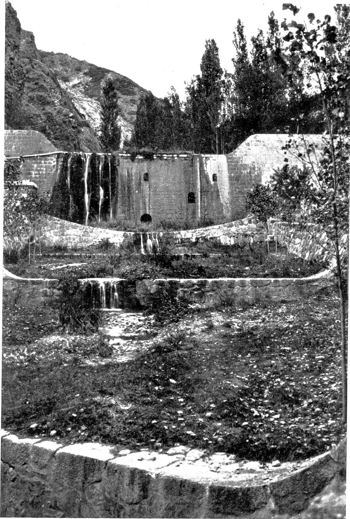
Abb. 5. Der Enseubach im Noguera-Pallaresatal Eine der höchsten und größten Retentionsperren im mittleren Lauf, mit Vorfperren
