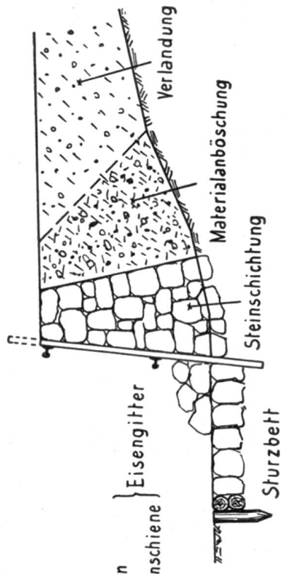
Längsschnitt
