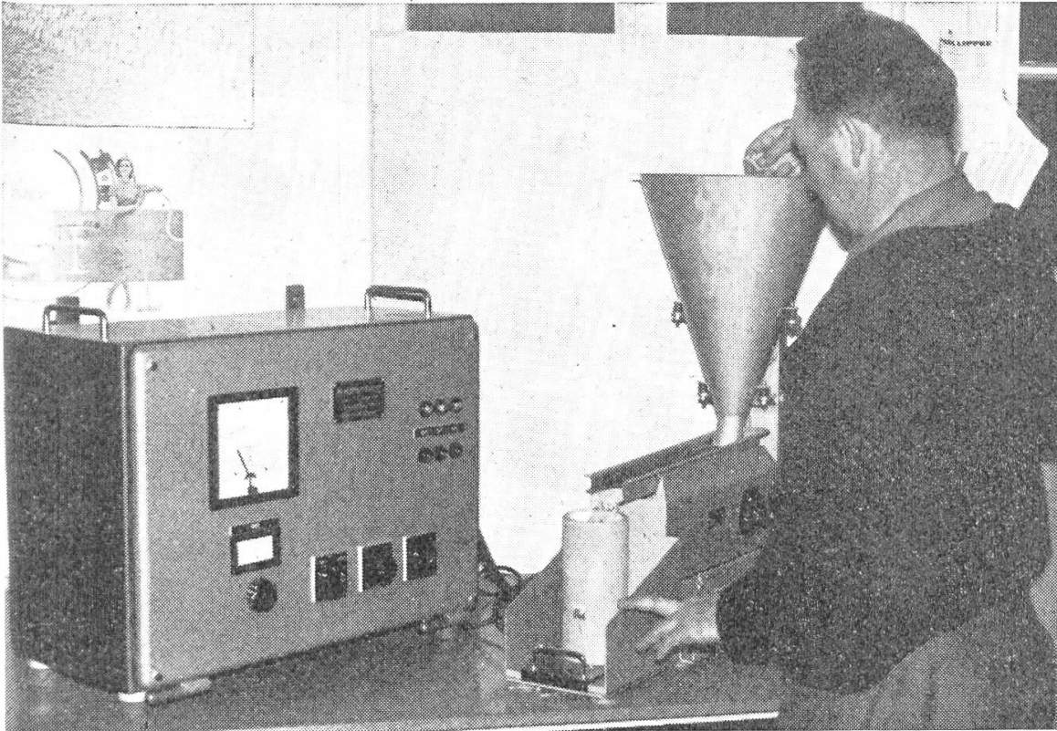
Fig. 10 DK-Meßgerät.
