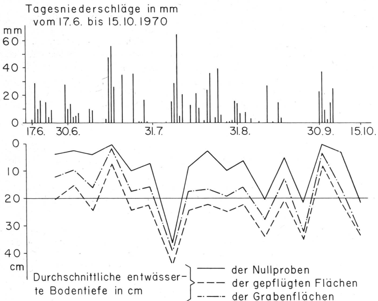
Abbildung 1. Wasserspiegellagen als Funktion der Zeit für drei verschiedene Behandlungsmethoden im Versuchsjahr 1970 und in der Versuchsfläche Hundschotten (Grabenentwässerung, Pflügen in Fallinie, unbehandelte Flächen).
