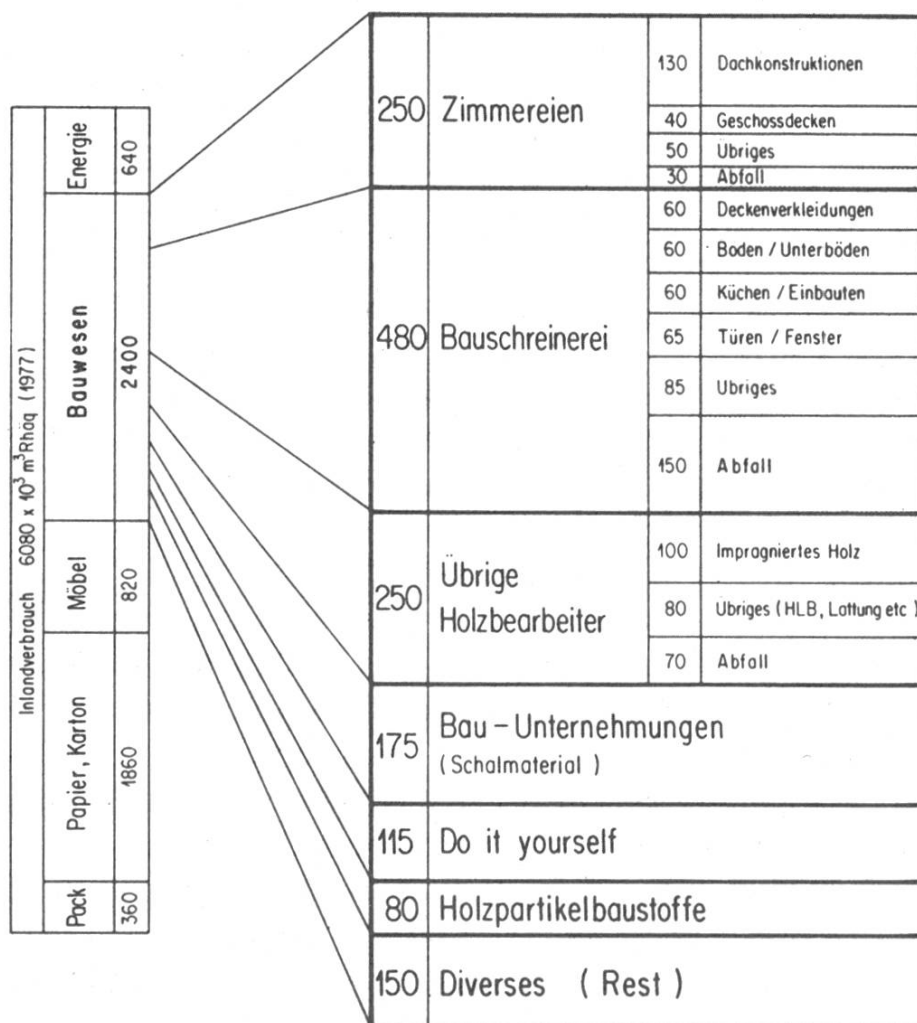
Abbildung 2. Holzfluss im Bauwesen (in 10^3 \text{ m}^3 fester Holzmasse, geschätzt aus Daten von 1977–80). Quelle: BNM Planconsult und EMPA. Anmerkung: Im linken Diagrammteil ist die Masseinheit 10^3 \text{ m}^3 \text{ Rhäq.}
