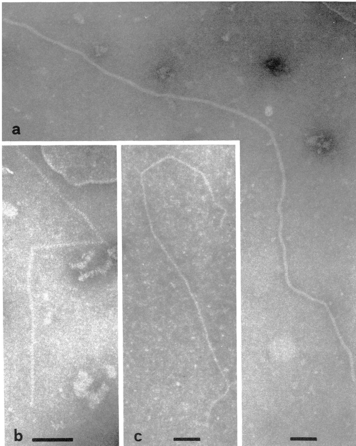
Abbildung 2. Elektronenmikroskopischer Vergleich closterovirusähnlicher Teilchen von Rebe und Fichte: a ) Closterovirusteilchen von Rebe mit Blattrollsymptomen; b ) und c ) closterovirusähnliche Teilchen von Fichte bei gleicher und stärkerer Vergrößerung (Balken = 100 nm).
