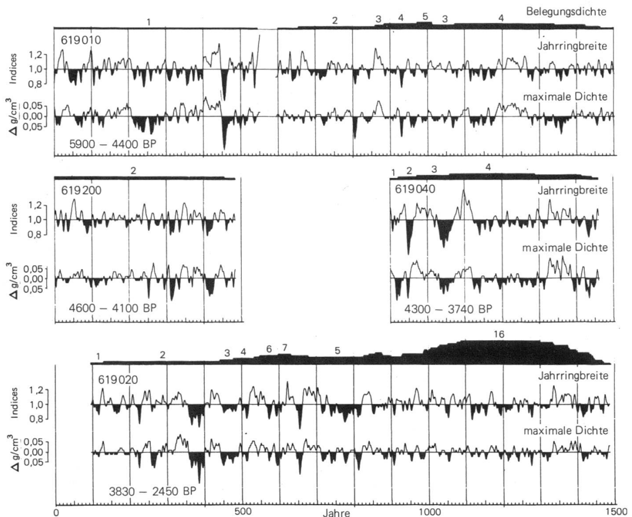
Abbildung 8. Vier längere Lärchenchronologien aus Grächen im zeitlichen Bereich von 5900 bis 2450 BP. Die Chronologien sind mit unkorrigierten Radiokarbonaten mit einer Genauigkeit von etwa 200 Jahren eingeordnet. Dargestellt sind die vom Alterstrend befreiten Mittelkurven der Jahrringbreiten und der maximalen Dichten mit den entsprechenden Belegungsdichten (oberste Balken). Die Kurven sind mit einem übergreifenden, gewichteten 13jährigen Filter (Low Julian) geglättet. Auffallend sind die grossen Variationen im kurz- und im mittelfristigen Bereich.
