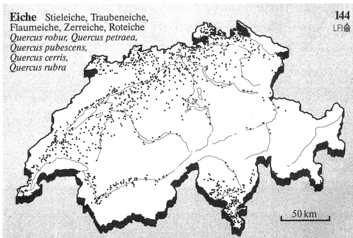
Abbildung 2. Verbreitungskarte Eiche.
