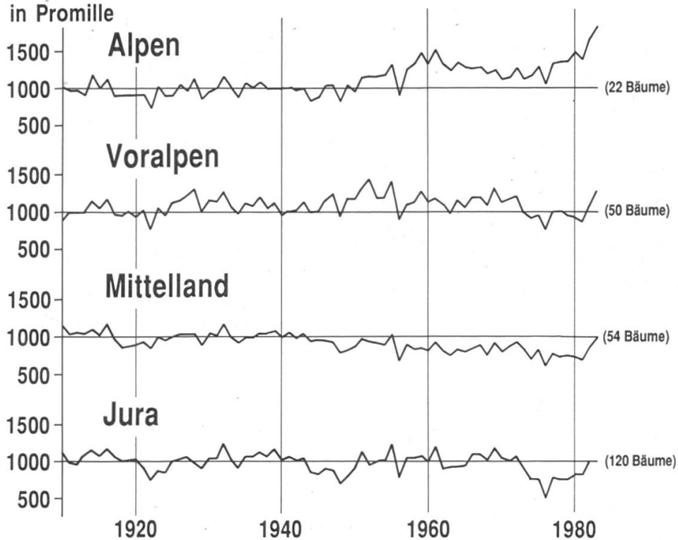
Abbildung 7. Mittlerer Zuwachsverlauf 1910 bis 1983 für Fichte und Tanne nach Regionen der Schweiz. Altersbereinigte Jahrringdaten von herrschenden und mitherrschenden, über 40 Jahre alten Bäumen. (Quelle: O.U. Bräker, briefl.)
