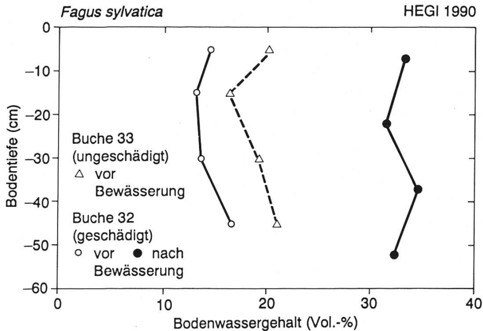
Abbildung 2. Die Tiefenabhängigkeit des Bodenwassergehaltes in rund 1 m Stammnähe der ungeschädigten Buche 33 (vor Bewässerung) und der geschädigten Buche 32 (vor und nach Bewässerung).
