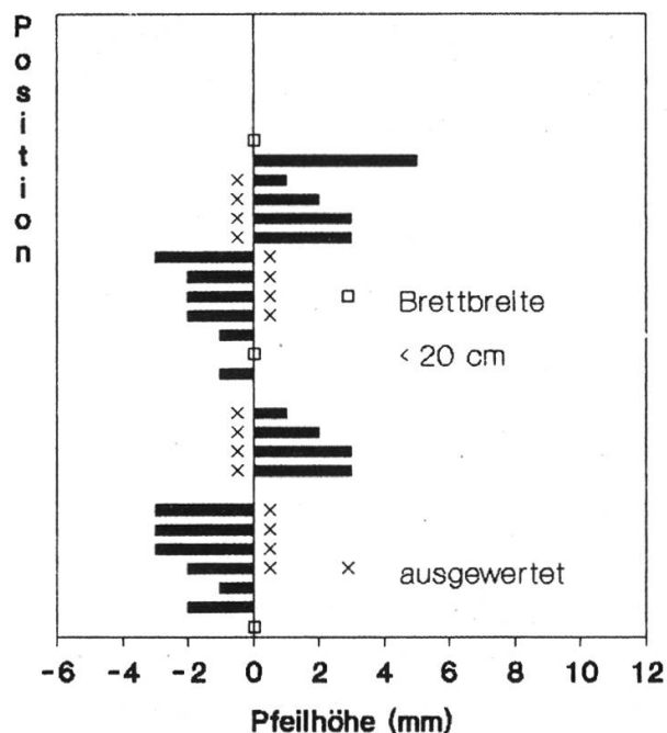
Werfen/Biegen: Pfeilhöhe über 20/100 cm
