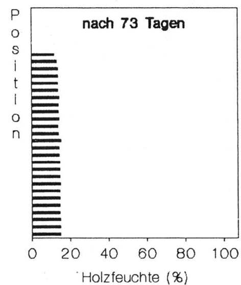
Abbildung 4. Holzfeuchte der Einzelbretter in der Stapelposition (Anordnung wie bei Blockware): Stapel I, halbseitig, zwei Bretterpakete übereinander.
