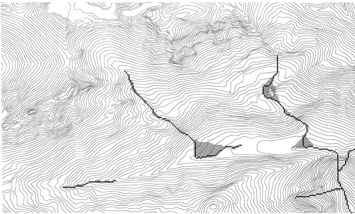
Abbildung 3. Reichweite und potentielle Ausbreitungsgebiete von Murgängen im Morgetebach (Gantrischgebiet, Berner Oberland). (Reproduktionsbewilligung der Landestopographie vom 25. Juli 1995.)
