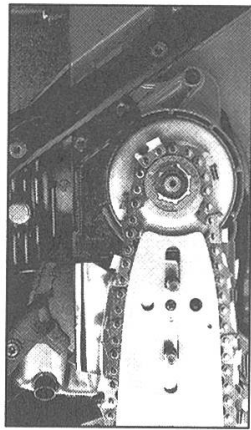
Innenliegende Kupplung Softstart
