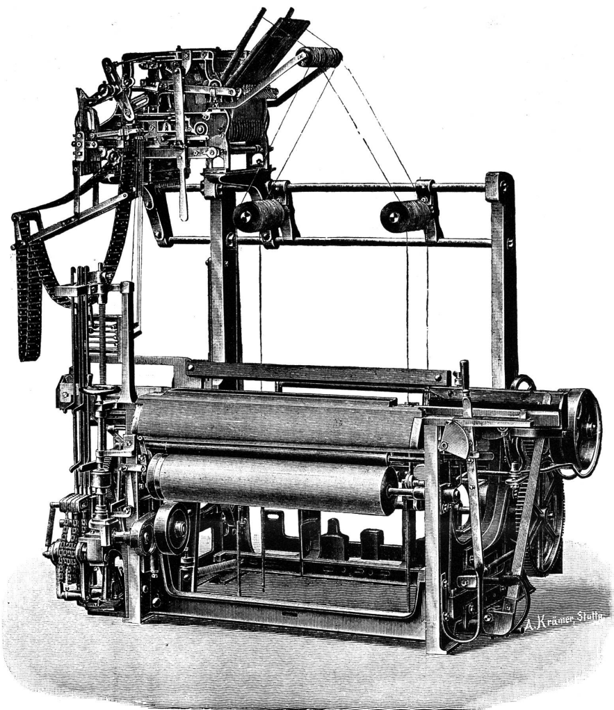
Seaton's automatischer Webstuhl.
