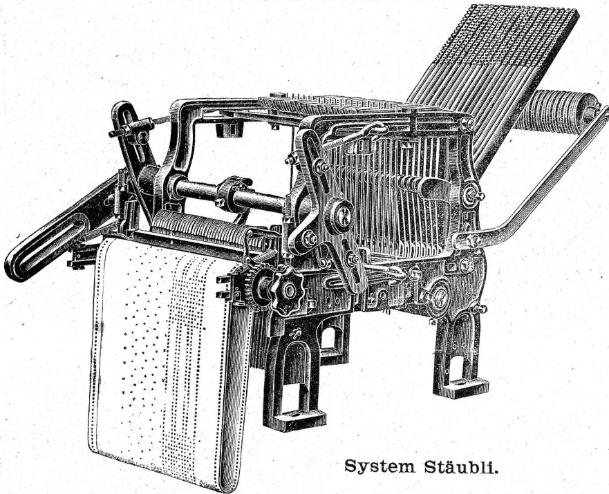
Schaffmaschine (Ratière) mit endlosem Papier-Dessin von 12–32 Schäfte.
