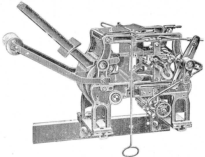
2 cylindrige Schaftmaschine
