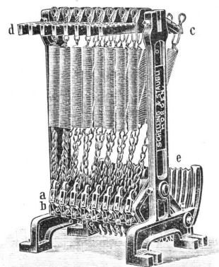
Federzugregister
