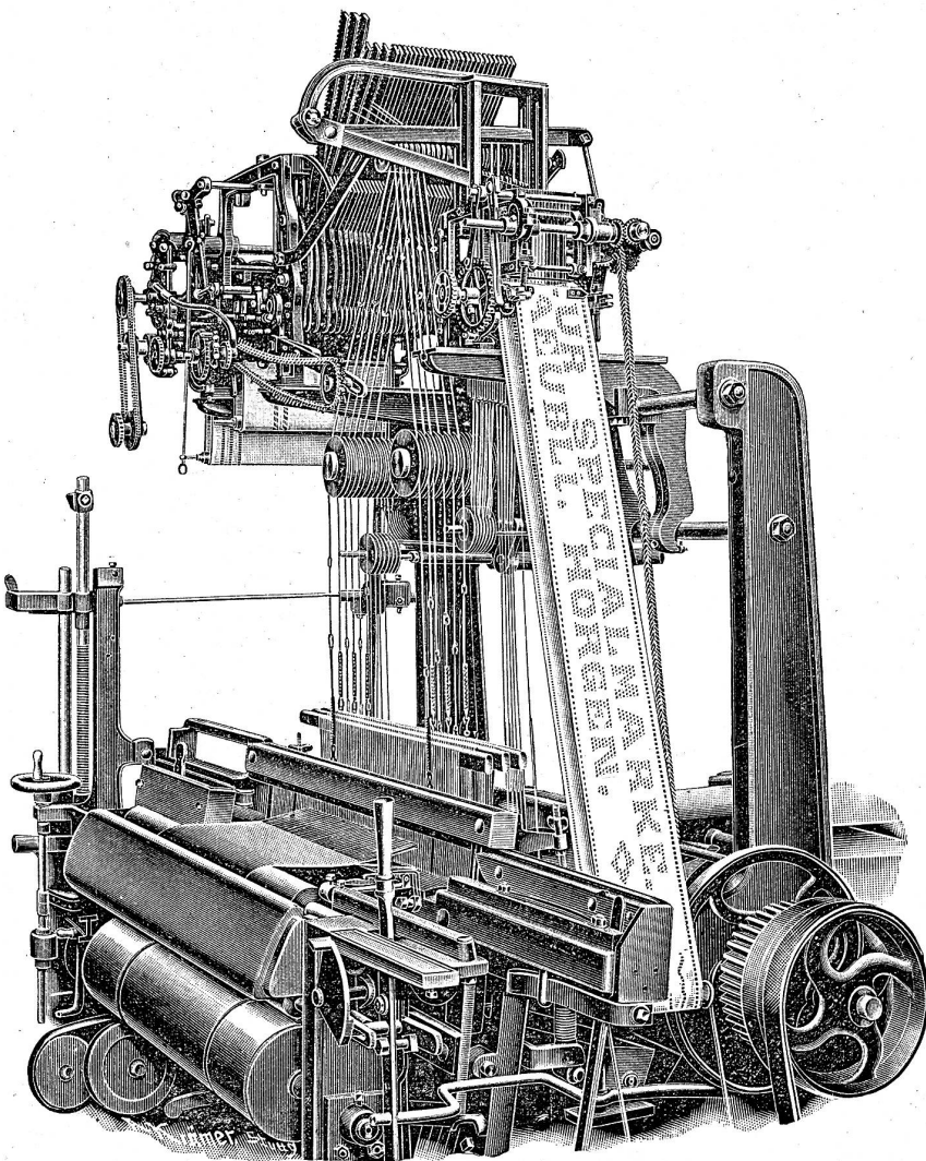
Fig. 3. Schaftmaschine für Namenweberei auf Rütli-Seidenstuhl montiert neben einer Schaftmaschine.
