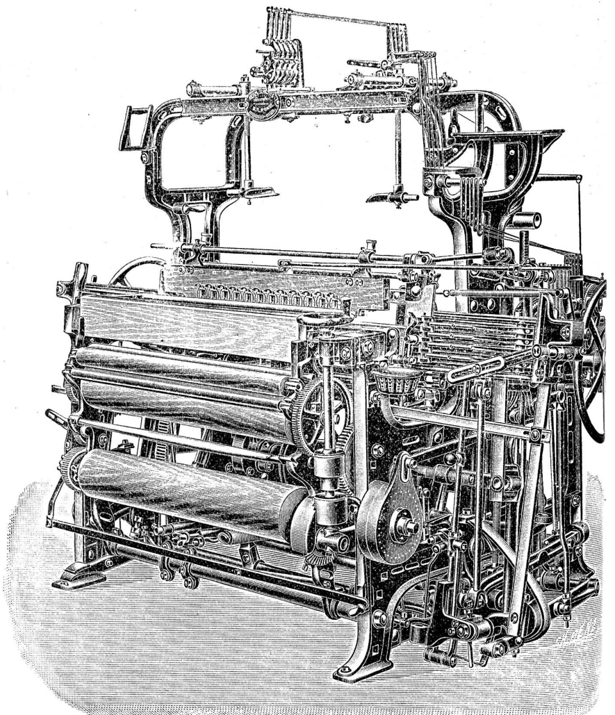
Brochier-Wechsel-(Lancier-) Webstuhl.
