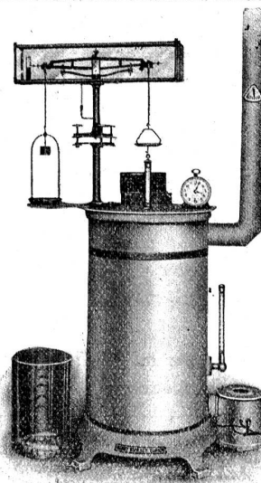
Gangharste Grösse: Für Versuche bis 500 gr. und mehr. Zur Bestimmung des Feuchtigkeitsgehaltes loser Textil-Rohstoffe und Garne von Wolle, Seide, Baumwolle, (Papier-Rohstoffe, Holzschliff etc.). Für Spiritus-, Gas- oder elektrische Heizung. Neueste solide Ausführung mit feinsten Präzisions- Wage in metallgefasstem Glasgehäuse, Drahtkorb, Hakenkranz, Thermometer, Wasserwage, Gewichtssatz
