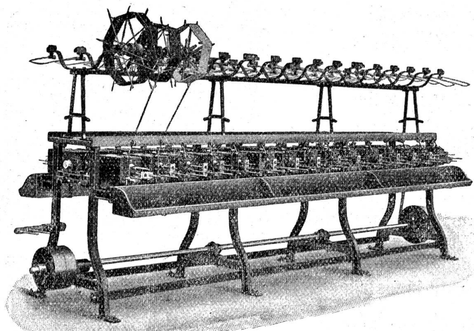
Kreuzschuss-Spulmaschine „Rapid“ direkt ab Strang arbeitend.
