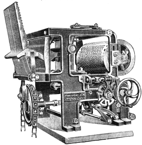
Doppelhub-Schäftmaschine „Reform“
