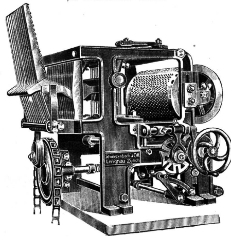
Doppelhub-Schaffmaschine „Reform“
