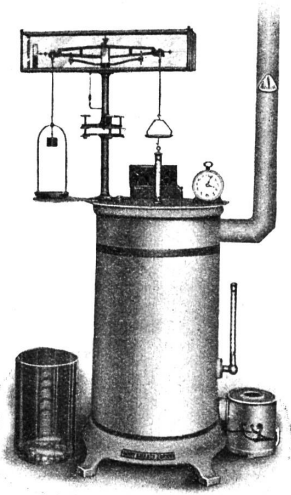
Gangbarste Grösse: Für Versuche bis 500 gr. und mehr. Zur Bestimmung des Feuchtigkeitsgehaltes loser Textil-Rohstoffe und Garne von Wolle, Seide, Baumwolle, (Papier-Rohstoffe, Holzschliff etc.). Für Spiritus-, Gas- oder elektrische Heizung. Neueste solide Ausführung mit feinsten Präzisions- Wage in metallgefasstem Glasgehäuse, Drahtkorb, Hakenkranz, Thermometer, Wasserwage, Gewichtssatz
