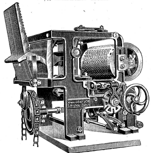
Doppelhub-Schaftmaschine „Reform“
