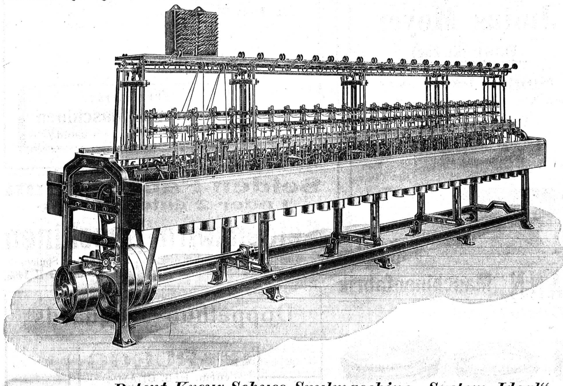
Patent-Kreuz-Schuss-Spulmaschine „System Ideal“
