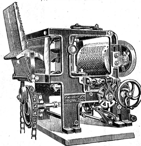
Doppelhub-Schaftmaschine „Reform“
