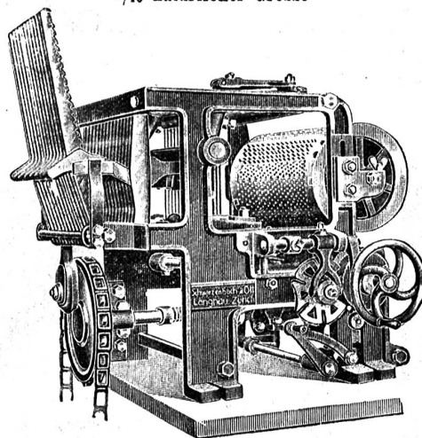
Doppelhub-Schaftmaschine „Reform“
