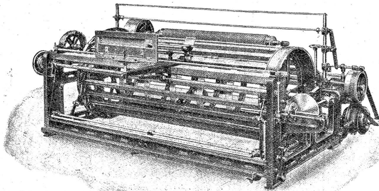
Unsere neueste komb. Seiden-Zettel- und Aufbaumaschine, unübertroffen in Bauart und Leistung
