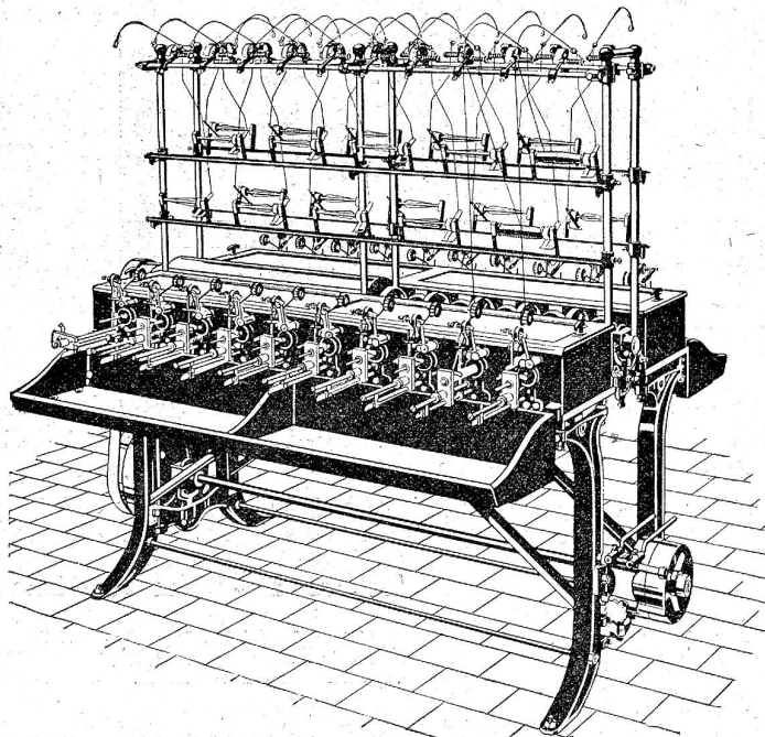
Kreuzschuß-Spülmaschine „Klein-Rapid“
