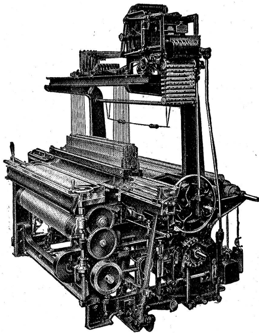
Neuer einseitiger 3-4 schütziger Seidenwebstuhl mit patentierter Wechsellvorrichtung für beliebige gerade Schußzahlen.
