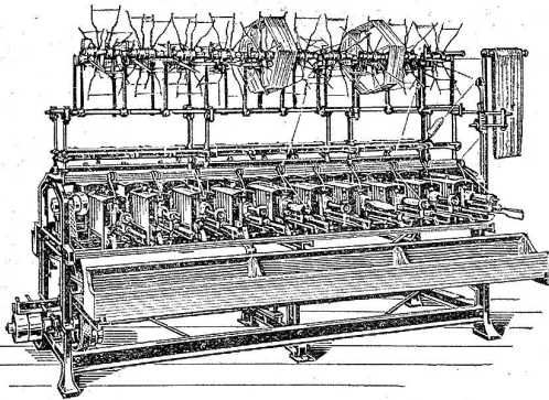
Kreuzschußspulmaschine „Produktiv CK“ Spulung ab Strang
