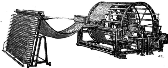
Kombinierte Seidenschner- und Aufbäummaschine, Modell mit großem Haspe
