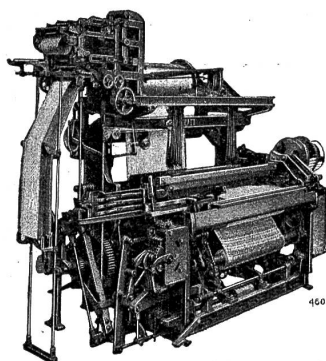
4-schütziger automatischer Webstuhl für Frottierwaren, Modell BAWF/4, kombiniert mit Rüti-Schaffmaschine
