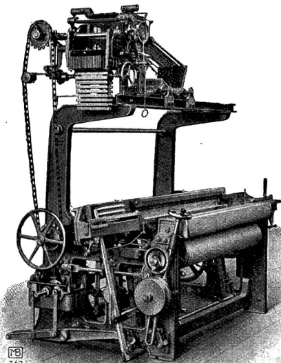
Vierschützig einseitiger Wechselstuhl
