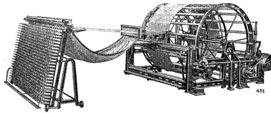
Kombinierte Seidenschere- und Aufbäummaschine, Modell mit großem Haspel
