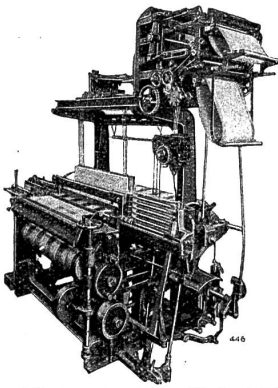
6-schütziger einseitiger Wechselstuhl mit direkter Stoffaufwicklung, Modell SDW/6, kombiniert mit RÜTI-Schaffmaschine
