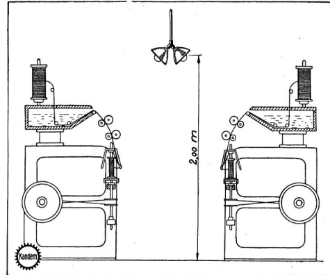
Abb. 9. Projektierungsbeispiel für zweckmäßige Beleuchtung von Naßspinnmaschinen.
