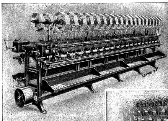
Pat. Spindellose Windmaschine Typ W. S.
