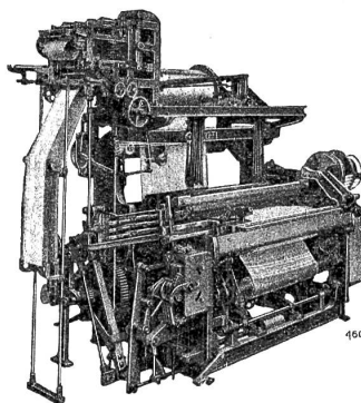
4-schütziger automatischer Webstuhl für Frottierwaren, Modell BAWF/4, kombiniert mit Rütli-Schaftmaschine
