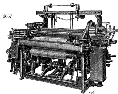
4-schütziger Webautomat Modell BAW 4, für Buntwaren
