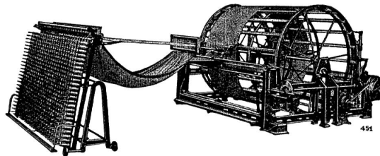
Kombinierte Seidenschär- und Aufbäummaschine, Modell mit großem Haspel
