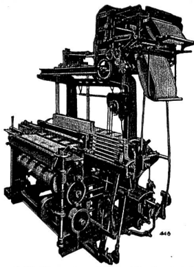
6-schütziger einseitiger Wechselstuhl mit direkter Stoffaufwicklung, Modell SDW/6, kombiniert mit RÜTI-Schaftmaschine
