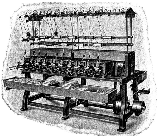
Kreuzschußpulmaschine Mod. CK 155
