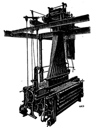
6-schütziger Spezialstuhl für Möbel- und Korsettsstoffe, Modell DWSC, kombiniert mit RÜTI-Jacquardmaschine
