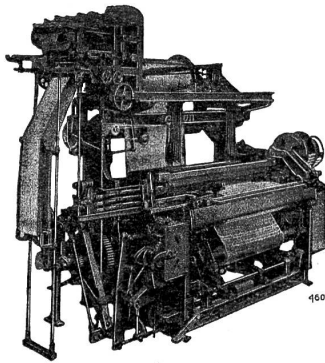
4-schütziger automatischer Webstuhl für Frottierwaren, Modell BAWF/4, kombiniert mit Rüti-Schaftmaschine
