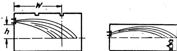
Abb. 8 und 9. Reich- oder Wurfweite und Gefälle des Luftstromes bei horizontalem und bei aufwärts gerichtetem Ausblas. h = Gefälle; W = Reichweite.
